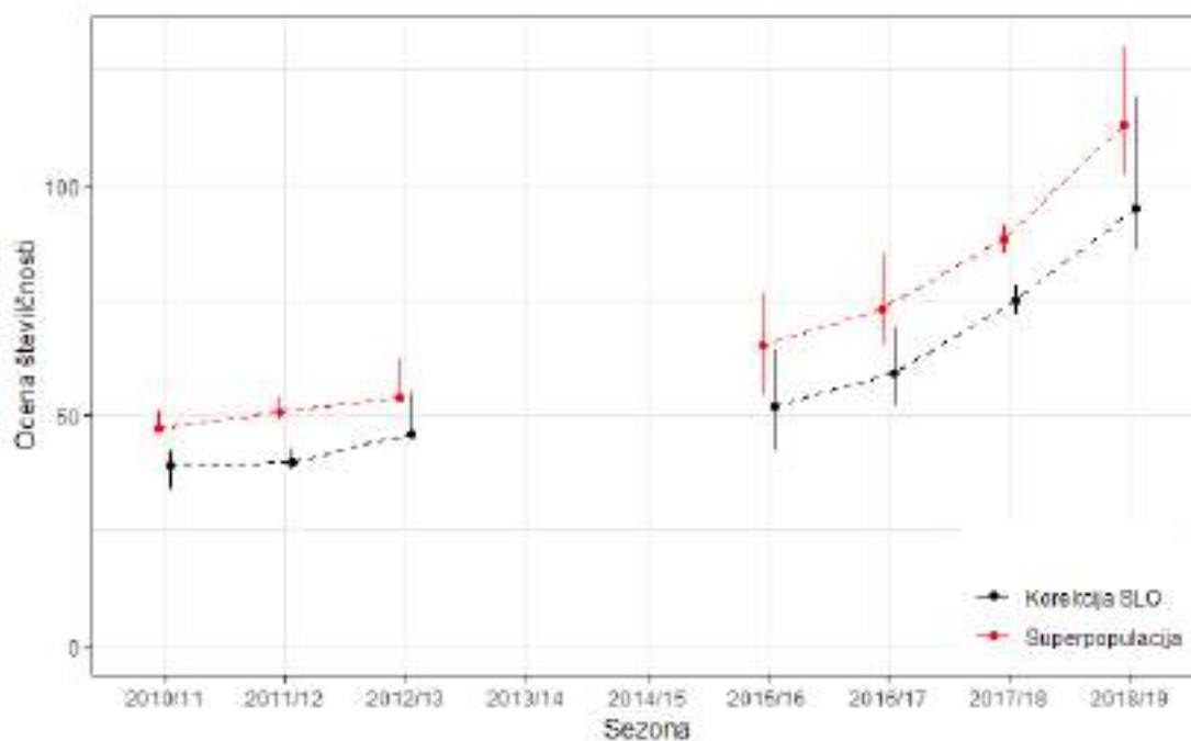
Slika 16: Večletna dinamika številčnosti populacije volkov v Sloveniji. Točke so srednje ocene, navpične črte kažejo 95 % interval zaupanja.
