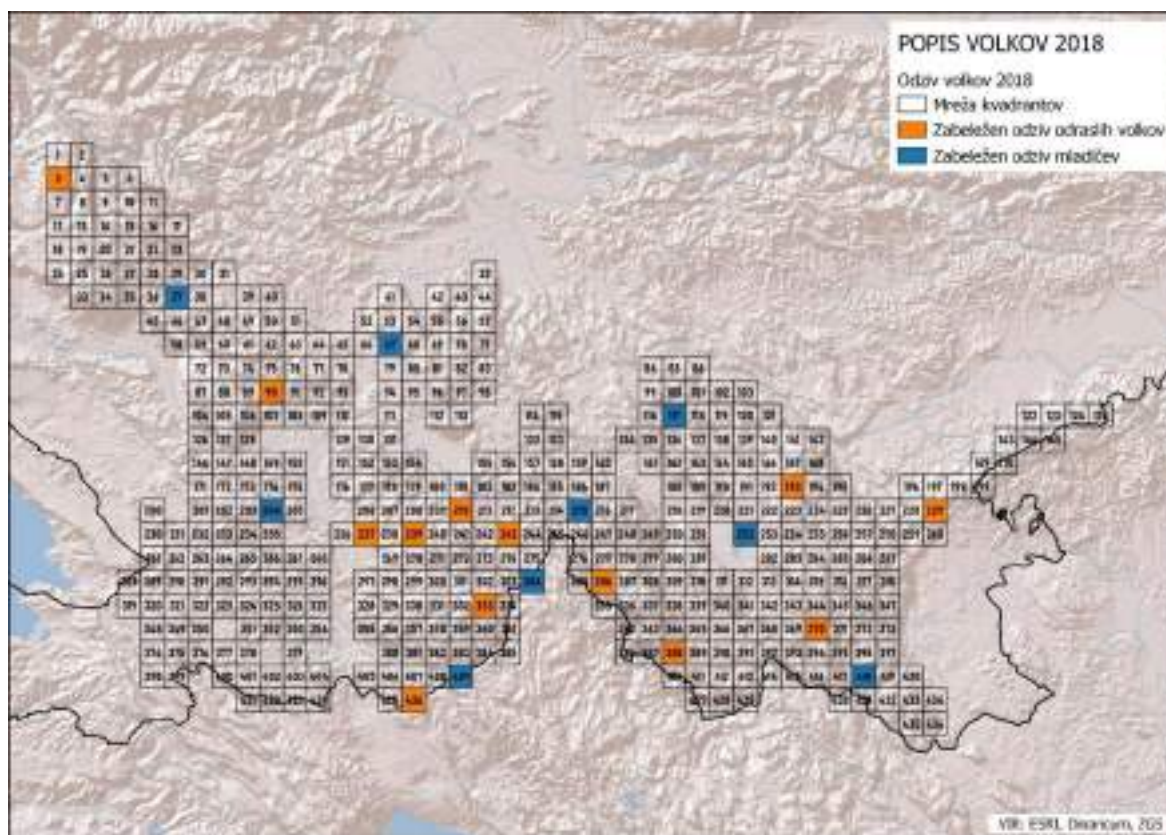
Slika 7: Mreža kvadrantov, v katerih je potekalo izzivanje oglašanja volkov v letu 2018, in zabeleženi odzivi volkov
