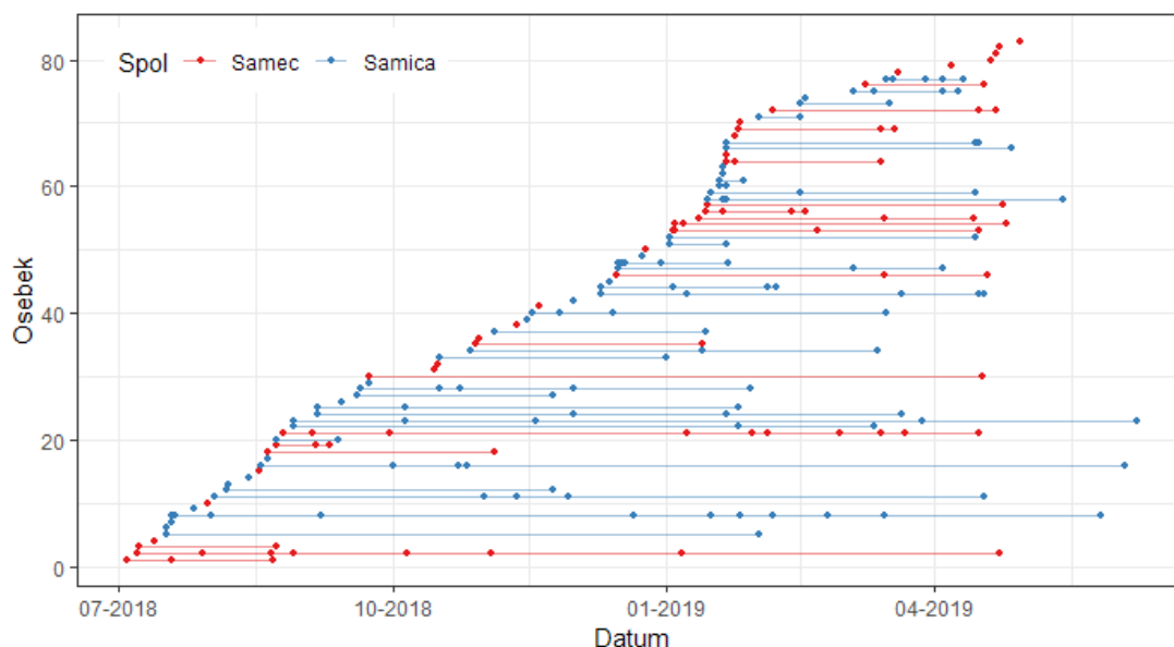
Slika 15: Saturacijski graf označevanja / ponovnega ulova za genetski monitoring volkov v Sloveniji v sezoni 2018/2019. Vsaka vodoravna črta je osebek, vsaka pika vzorec. Osebkam so kronološko razporejeni glede na prvi »ulov« (najdbo prvega vzorca).
