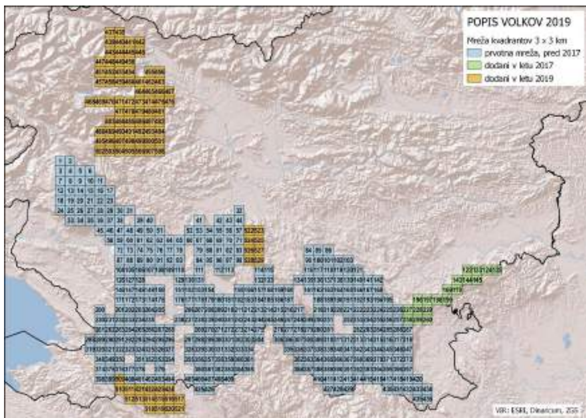
Slika 20: Mreža kvadrantov, po kateri se je v sezoni 2019/2020 izvajalo zvočno zaznavanje volkov s pomočjo izzivanja oglašanja
